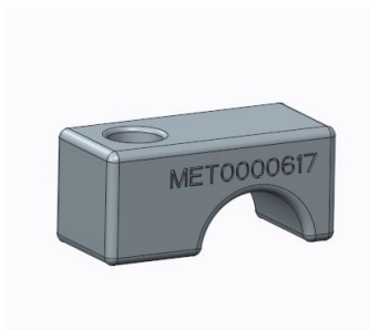
Universal Metercube Lid Clamp
